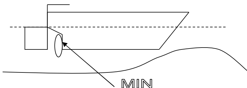
Рис. 4 «Явление просадки и прохождение перекатов»
