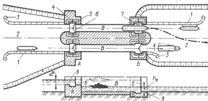
Рис.22. Шлюз:
