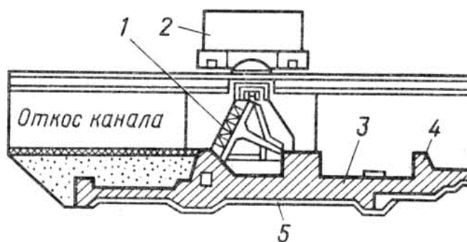
Рис.26. Аварийные ворота канала:
